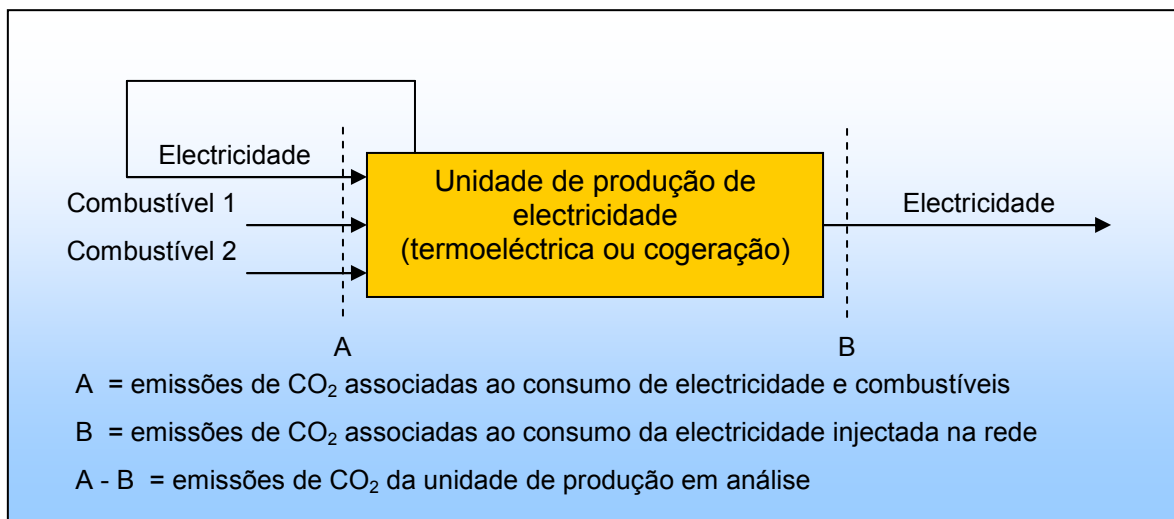
Figura 2 – Metodologia de contabilização de emissões de unidades de produção de electricidade
